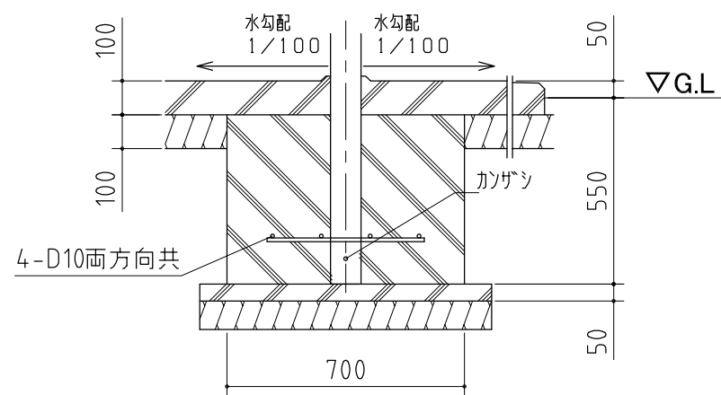
A-A' 断面 1/20
